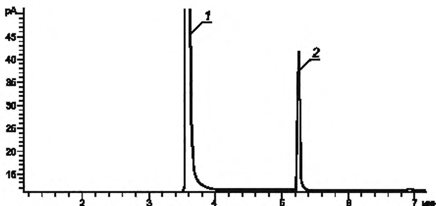
1 — этиловый спирт, 2 — кротоновый альдегид
