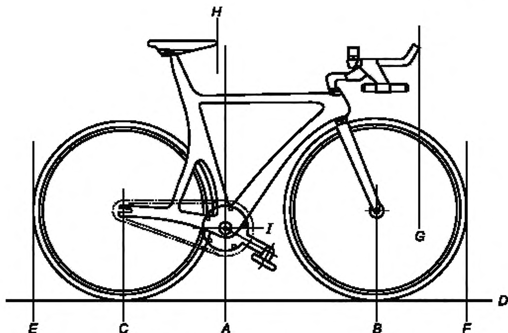
Рисунок 1 — Основные параметры и размеры велосипеда
