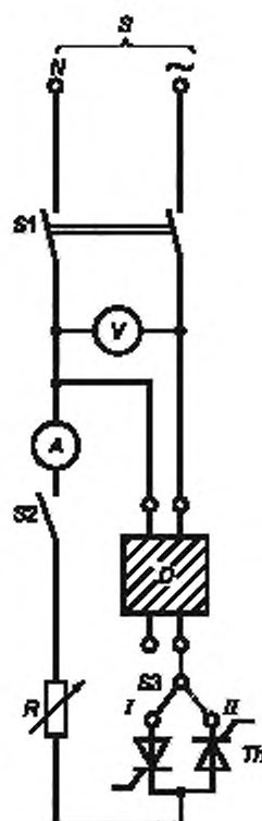
S — источник электрической энергии; V — вольтметр; A — амперметр, показывающий среднее квадратическое значение; D — испытуемое УЗО-ДП, R — регулируемый резистор; Тл — тиристор; S1 — двухполюсный выключатель; S2 — однополюсный выключатель; S3 — однополюсный выключатель на два направления
