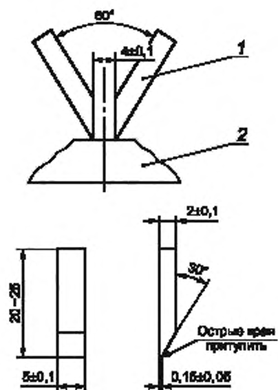
1 — электрод, 2 — образец
