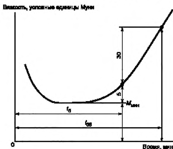
Рисунок 4 — Типичная кривая характеристик подвулканизации при использовании большого ротора
