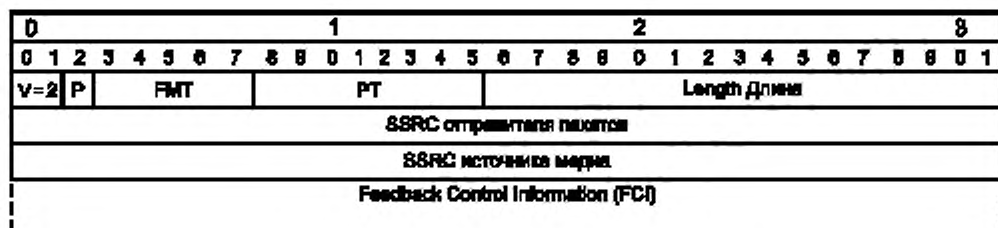
Рисунок В.4 — Формат пакета сообщения FB RTCP
