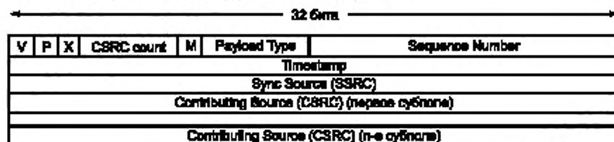
Рисунок 11 — Формат заголовка протокола RTP
