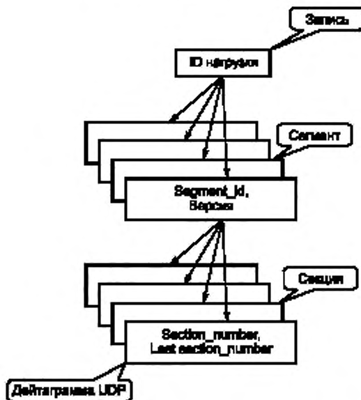
Рисунок 9 — Взаимосвязь между секциями, сегментами и записями
