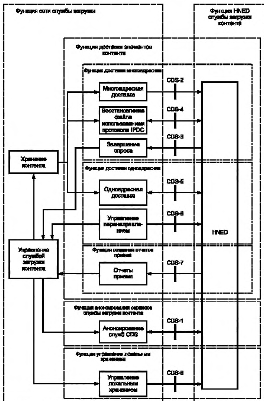
Рисунок 13 — Эталонная структура службы загрузки контента
