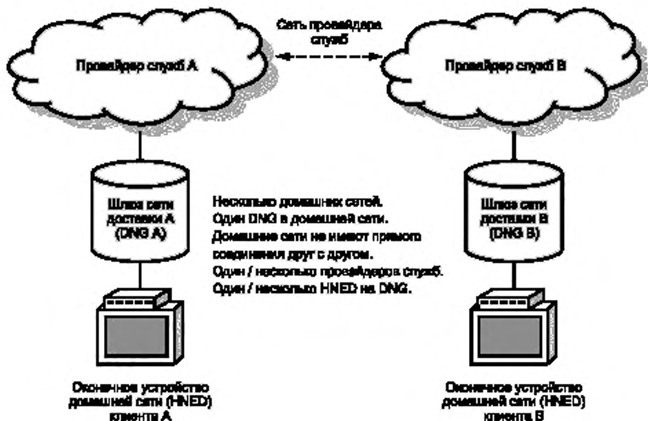
Рисунок 5 — Множество домашних сетей (сложная домашняя сеть)
