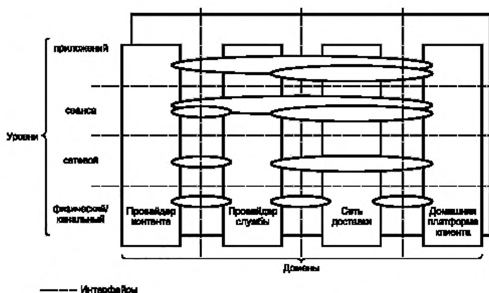
Рисунок 1 — Модель уровней DVB-IP
