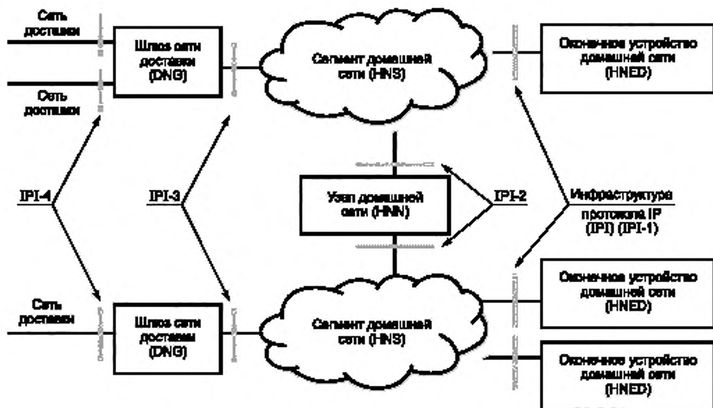
Рисунок 2 — Эталонная модель домашней сети
