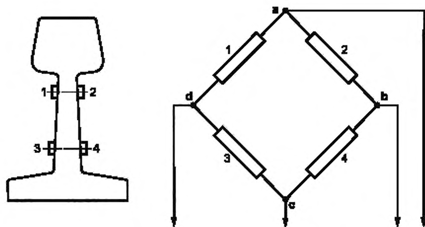
Точки а и с — измерительная диагональ; d, b — питание моста
