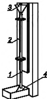
1 — стеклянная трубка; 2 — штатив; 3 — конусообразная воронка; 4 — ящик
