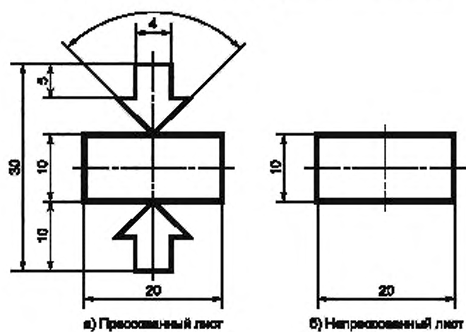
Рисунок Г.1 — Размеры символического изображения типа листов
