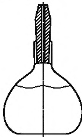
Рисунок 2 — Стеклоанный пикнометр типа Гей-Люссака
