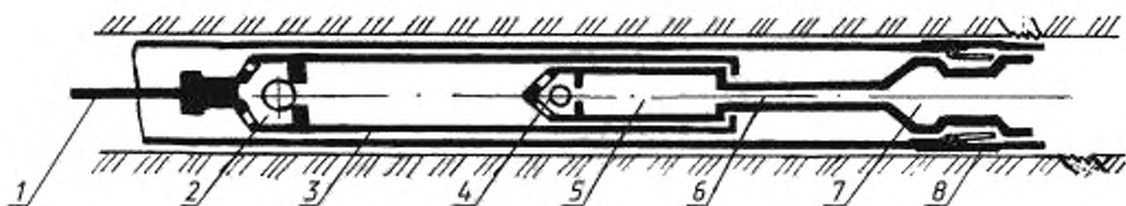
1 — шток; 2 — нагнетательный клапан; 3 — цилиндр; 4 — всасывающий клапан; 5 — плунжер, 6 — патрубок-удлинитель. 7 — упорный ниппель с конусом; 8 — насосно-компрессорная труба с замковой опорой
