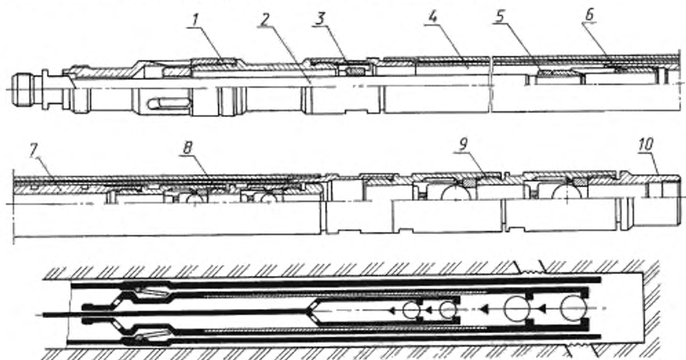
Рисунок 1 — Схема насоса типа НВ1С
