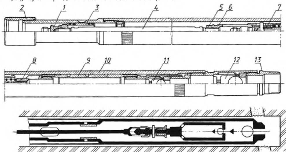
Рисунок 11 — Схема насоса типа ННАБ
