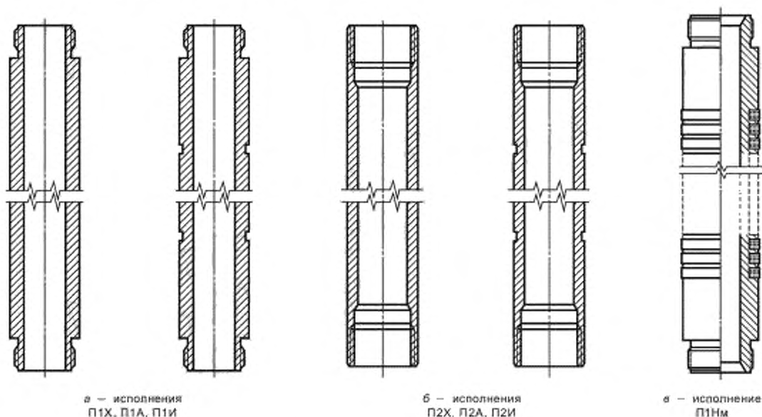
Рисунок 15 — Плунжеры
