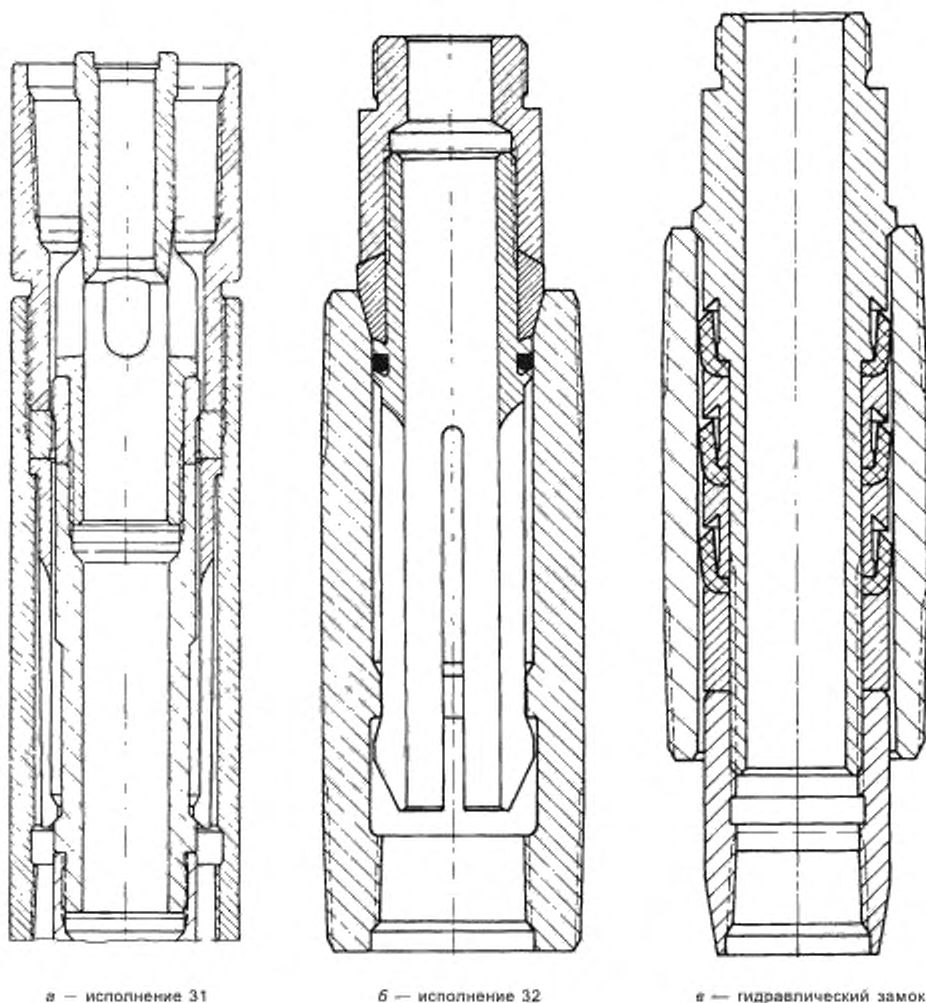
Рисунок 17 — Замки
