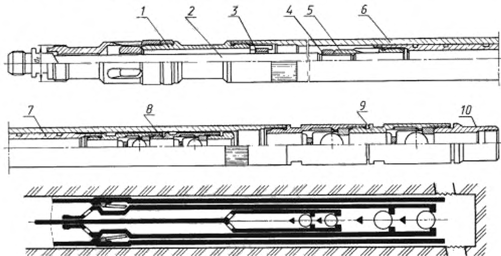
Рисунок 2 — Схема насоса типа НВ1Б
