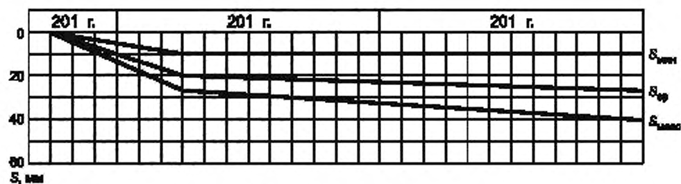
Рисунок Г.4 — График развития перемещений
