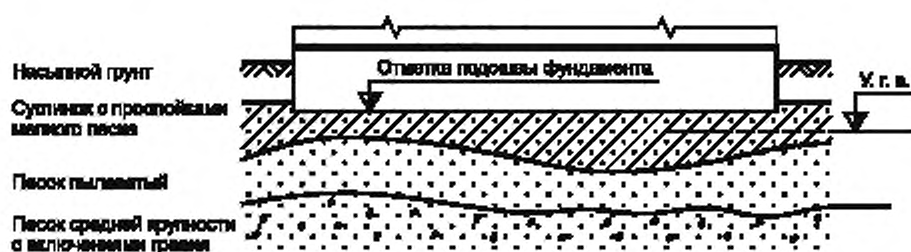
Рисунок Г.1 — Схема фундамента и основания
