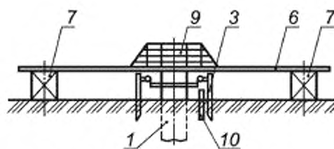
в) Установка с тарированным грузом
