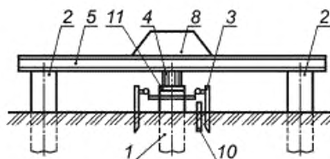
г) Установка комбинированная
