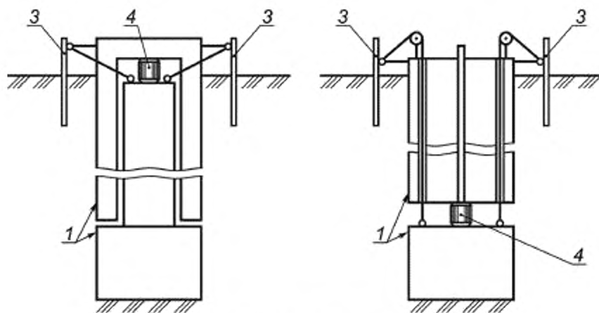
ж) Схемы установок с самоанкерующимися сваями-штампами
