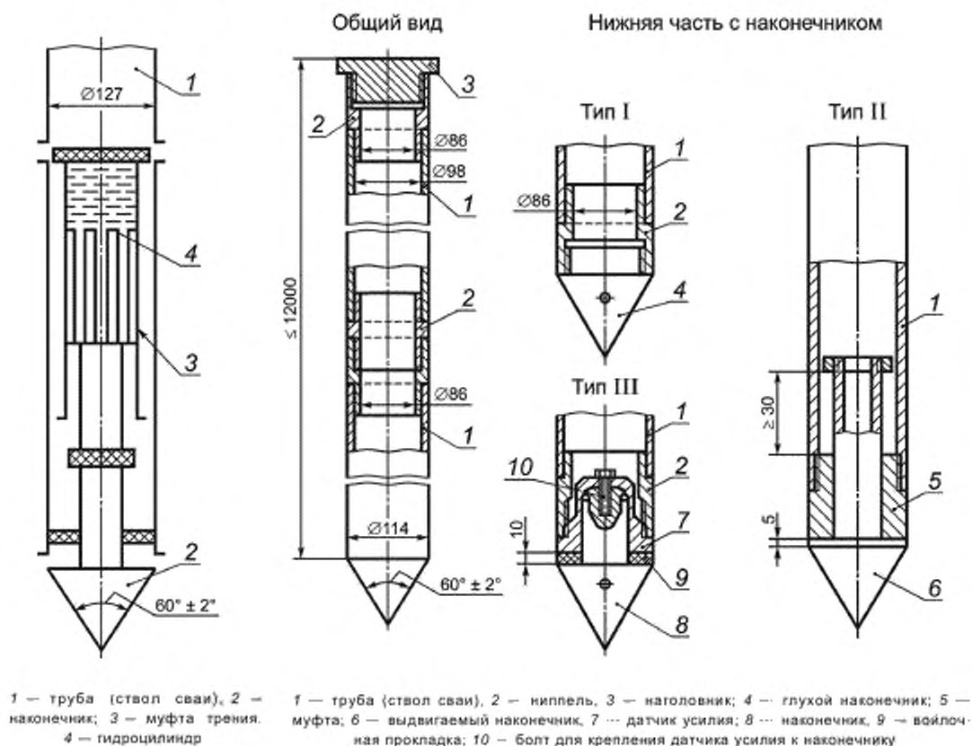
Рисунок В.1 — Схема конструкции сваи-зонда
