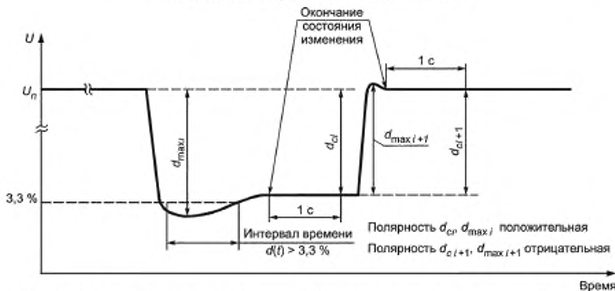
Рисунок В.2д — Пример для объяснения последовательности и полярности d_{\max} и d_c при многократных установившихся состояниях
