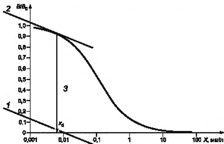
Рисунок 6 — Полулогарифмический график кривой B/B_0 для конкурентного иммуоферментного анализа ELISA 17-гидроксипрогестерона
