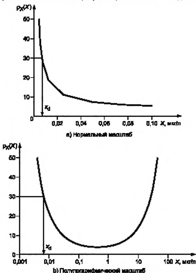
Рисунок 5 — Коэффициент вариации приведенной переменной состояния p_X(X) (функция прецизионности) и минимальное обнаруживаемое значение x_d в нормальном и полулогарифмическом масштабе для конкурентного иммуноферментного анализа ELISA
