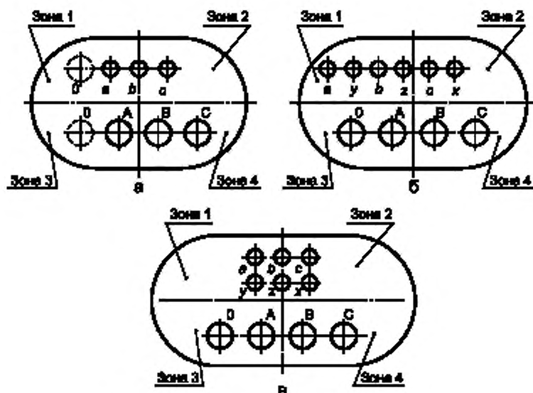
Рисунок 1 — Двухобмоточные трансформаторы
