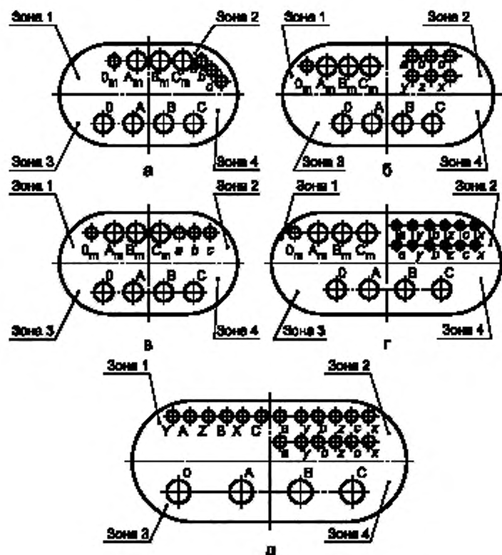
Рисунок 3 — Трехобмоточные трансформаторы
