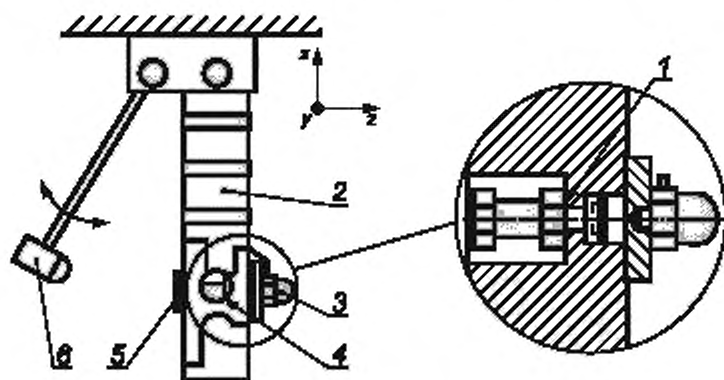
1 — измерительная поверхность, использованная при первичной калибровке; 2 — маятник-наковальня; 3 — калибруемый преобразователь; 4 — эталонный преобразователь; 5 — бутиленовый каучук; 6 — маятник-молоток
