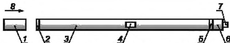
Рисунок 7 — Схема калибратора удара с разрезным стержнем Гопкинсона
