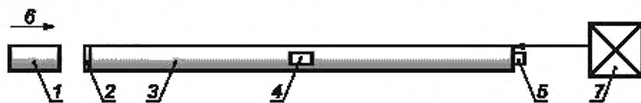
Рисунок 6 — Схема калибратора удара со стержнем Гопкинсона
