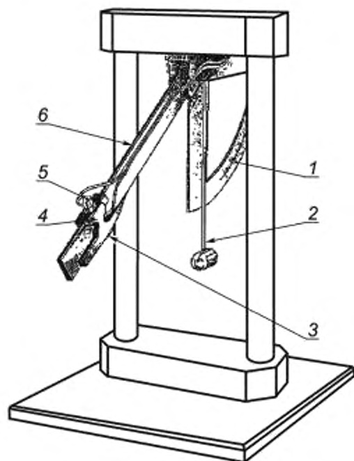
1 — шкала с регулируемым углом; 2 — маятник-молоток; 3 — упругая прокладка; 4 — эталонный преобразователь; 5 — калибруемый преобразователь; 6 — маятник-наковальня
