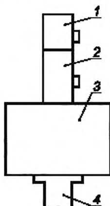
1 — калибруемый преобразователь; 2 — эталонный преобразователь; 3 — сейсмическая масса; 4 — наковальня
