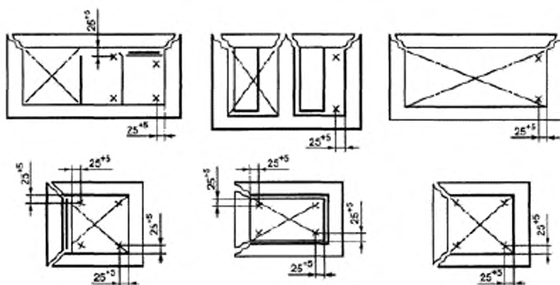
Рисунок Д.1 — Схемы расстановки термодатчиков в объеме сейфа
