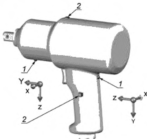
1 — предпочтительная точка измерений, 2 — дополнительная точка измерений
