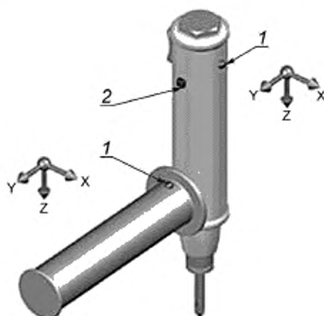
Рисунок 17 — Точки и направления измерений для шуруповерта с поддерживающей рукояткой
