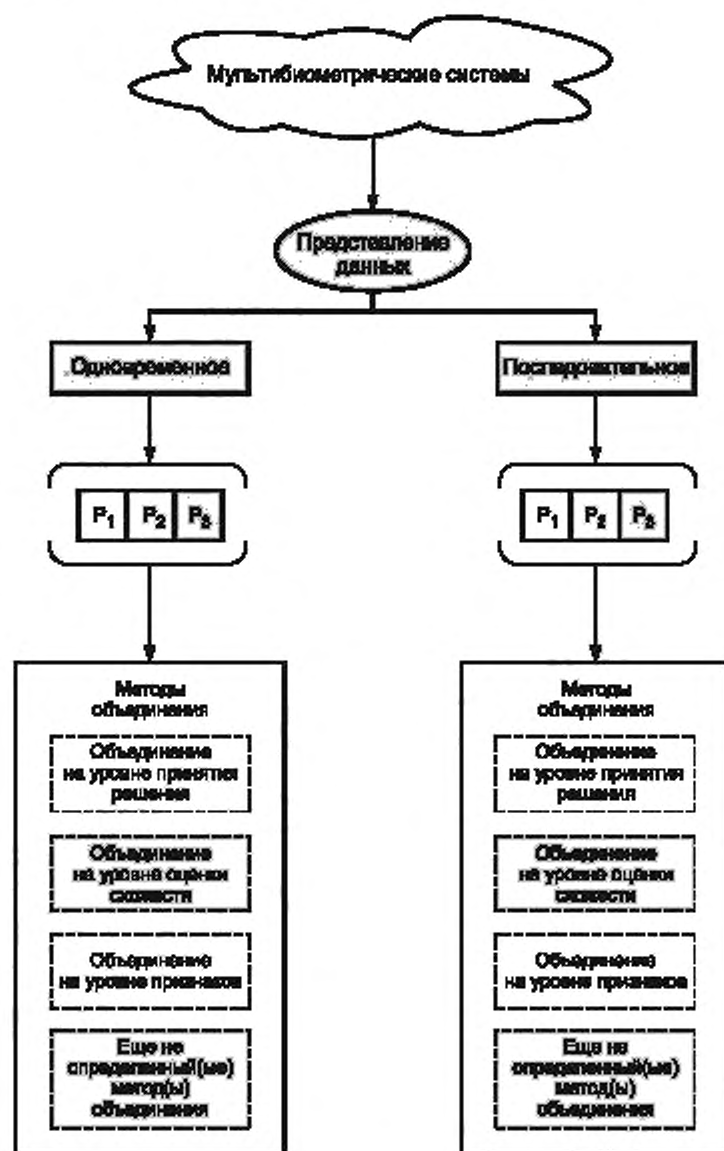
Рисунок 1 — Модель мультибиометрической системы
