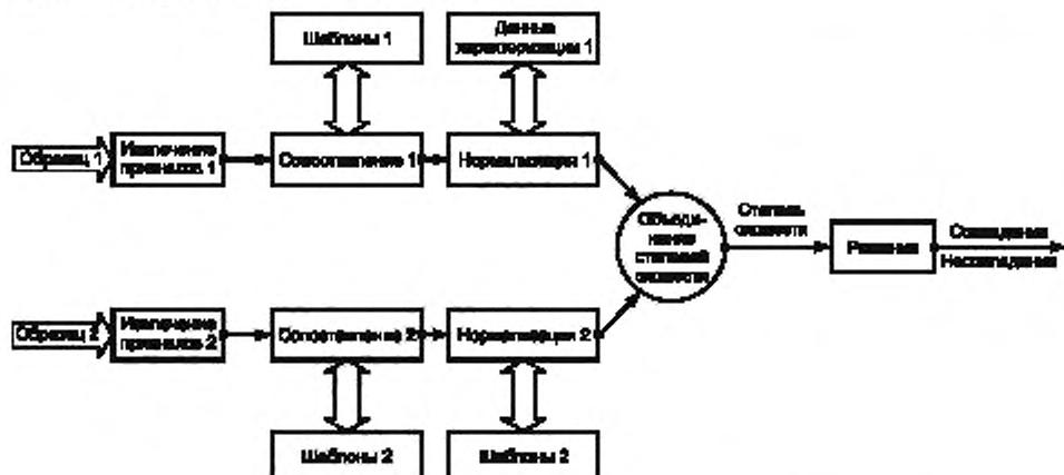
Рисунок 5 — Структура объединения на уровне степеней схожести
