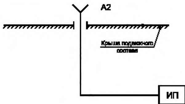
Рисунок ДА.1 — Схема измерения напряжения электромагнитных помех, создаваемых подвижным составом в канале железнодорожной радиосвязи гектометрового радиочастотного диапазона
