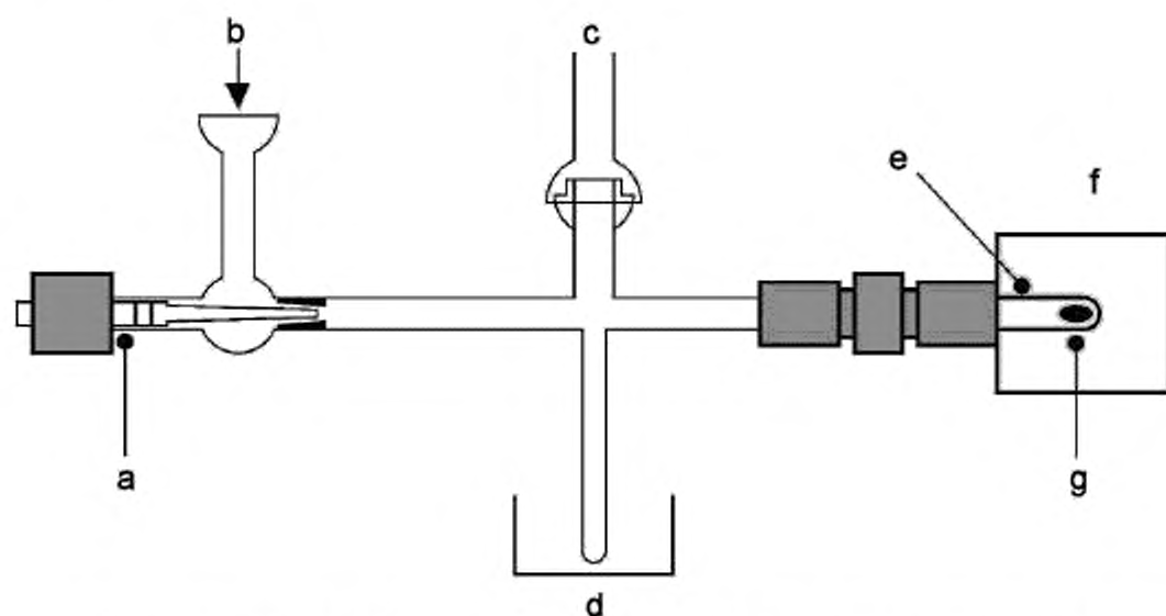
Рисунок В.2 – Установка для графитизации
