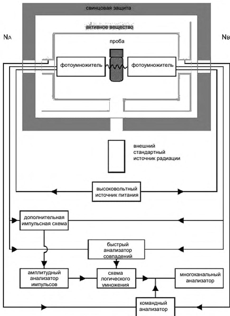
Рисунок А.1 – Жидкостный сцинтилляционный счетчик
