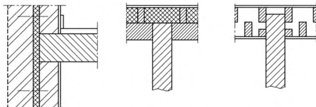
Рисунок E.4 – Примеры жесткого T-образного соединения
