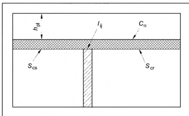
Рисунок Ф.1 – Величины для определения косвенной воздушной звукопередачи
