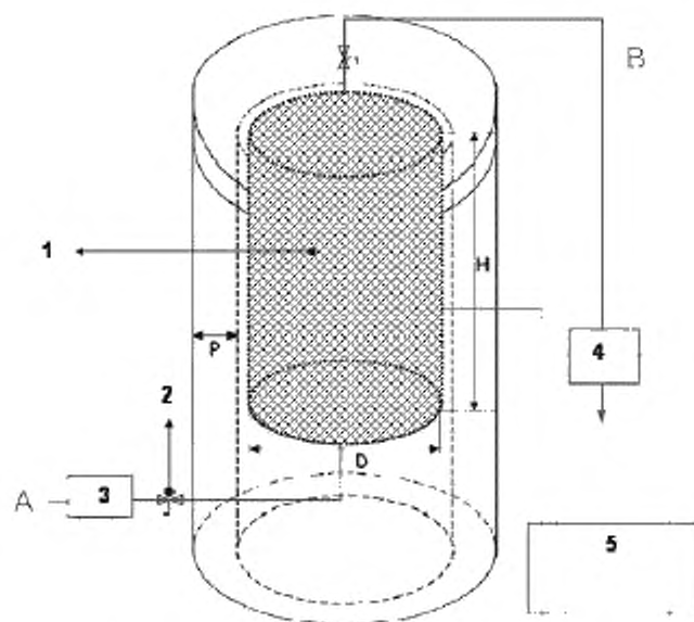
1 – контейнер с твердым топливом из бытовых отходов; D – внутренний диаметр реактора, H – внутренняя высота реактора; H/D = 1,465 \pm 0,080 ; P – толщина внешних стенок реактора = 70 \pm 5 мм. – клапан проверки герметичности системы реактора; 2 – регуляторы расхода и расходомеры; 3 – воздушный насос с датчиком температуры воздуха на входе; 4 – система определения содержания кислорода в выхлопном воздухе; 5 – система сбора данных; A – воздухоприемник; B – выходной поток воздуха.
