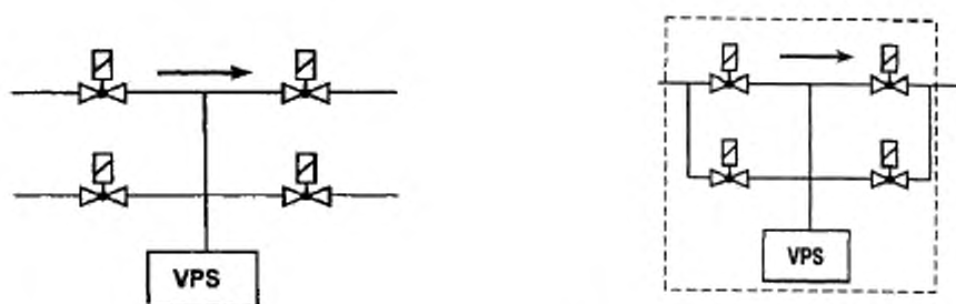
б – пример системы VPS с интегрированными клапанами
