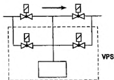
с — пример системы VPS с частично интегрированными клапанами
