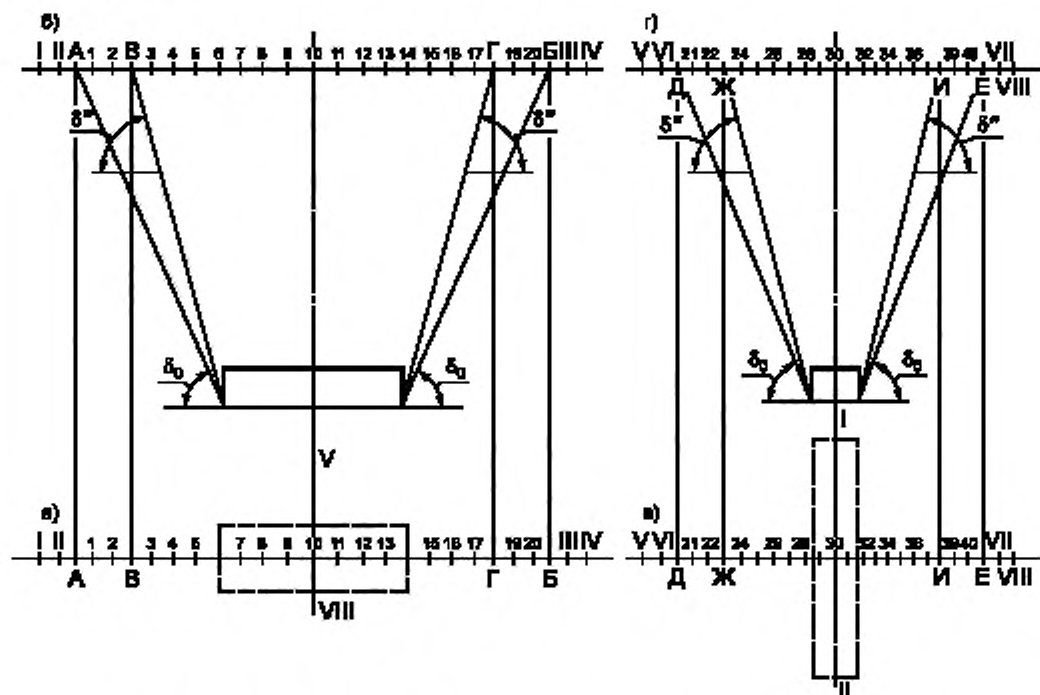
а) и б) — на плане и разрезе вдоль сооружения; а) и г) — на плане и разрезе поперек сооружения, I, II, III, IV, V, VI, VII, VIII — опорные реперы; 1—40 — рабочие реперы; АБ и ДЕ — зоны влияния подземного сооружения на земную поверхность; ВГ и ЖИ — зоны возможного образования трещин
