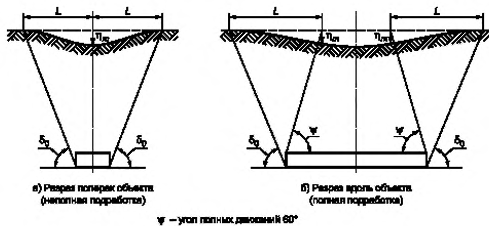
Рисунок Р.1 — Основные параметры мурды сдвижения
