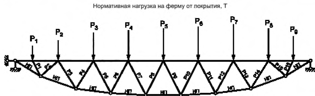
Рисунок К.1 — Расчетная схема деревометаллической фермы покрытия Крытого конькобежного центра
