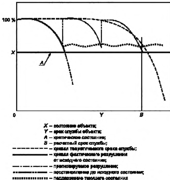
Рисунок A.2 — Стандартные циклы ремонта в течение срока службы объекта, подвергнутого разрушению
