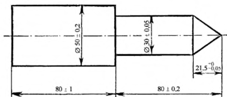
Рисунок 3 – Испытательный щуп
