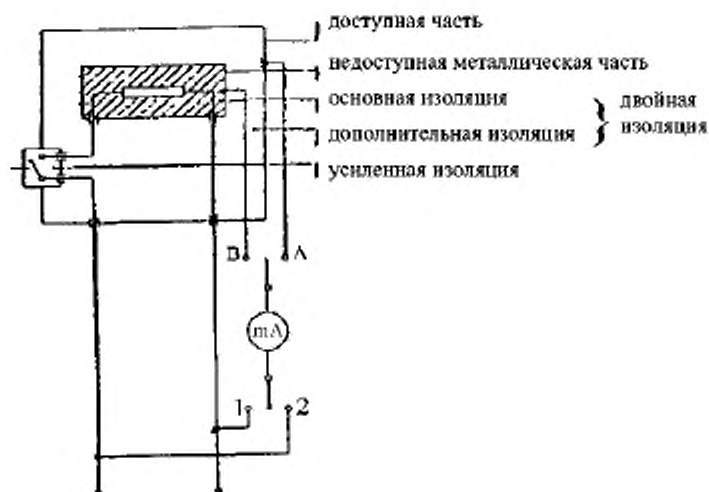
Рисунок 4 – Схема измерения тока утечки при рабочей температуре для однофазных приборов класса II
