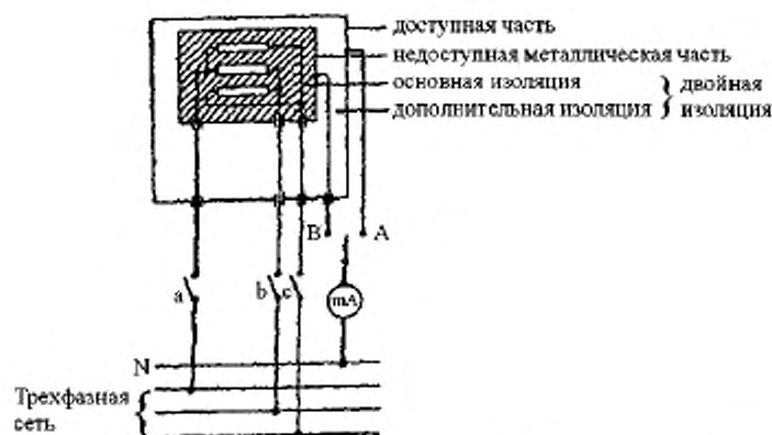
Рисунок 6 – Схема измерения тока утечки при рабочей температуре для трехфазных приборов класса II
