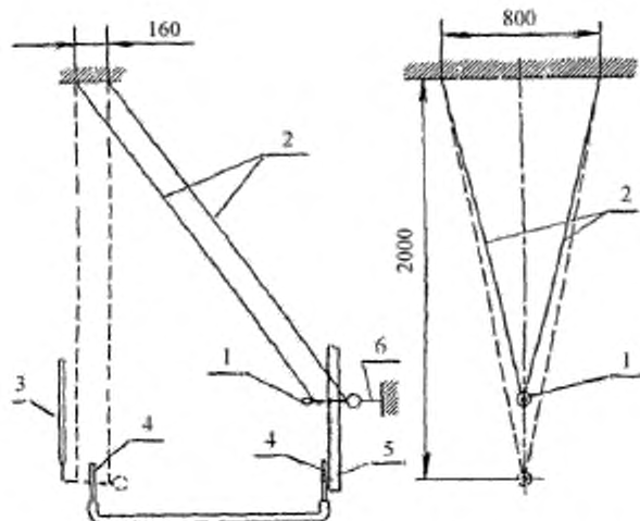
Рисунок R.6 – Установка для настройки калибрующего устройства
