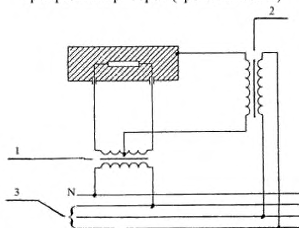
1 – разделительный трансформатор; 2 – повышающий трансформатор; 3 – трехфазная сеть
