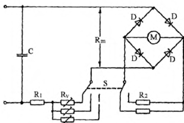
Рисунок G.1 – Схема цепи для измерения тока утечки
