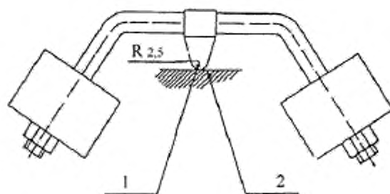
Рисунок 12 – Устройство для вдавливания шарика
