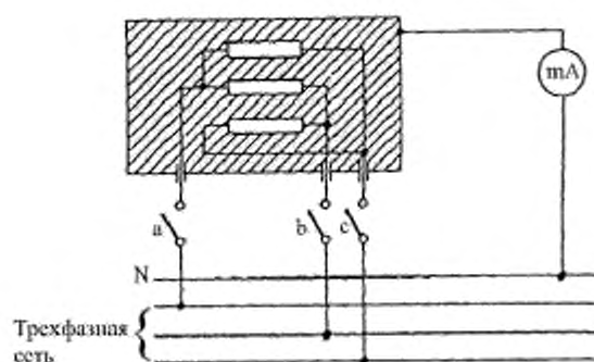
Рисунок 7 – Схема измерения тока утечки при рабочей температуре для других трехфазных приборов (кроме класса II)
