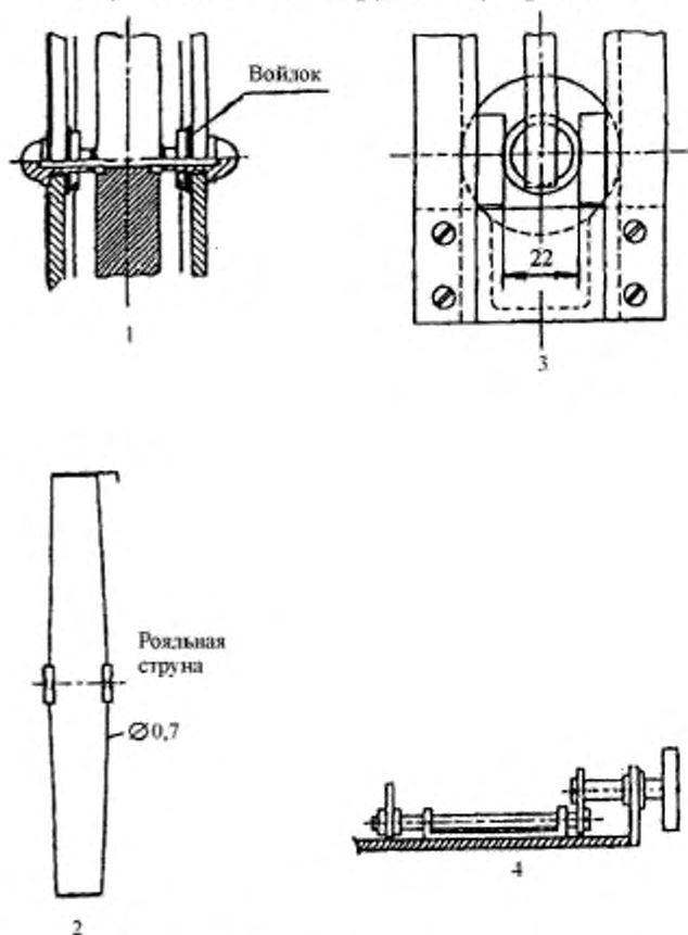
Рисунок R.5 – Детали калибрующего устройства
