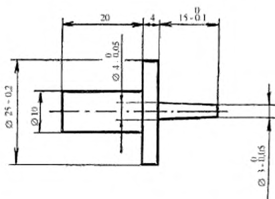
Рисунок 2 – Испытательный стержень
