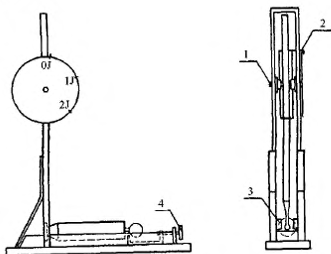
1 – подшипник; 2 – фиксирующий указатель; 3 – спусковое основание; 4 – спусковой механизм
