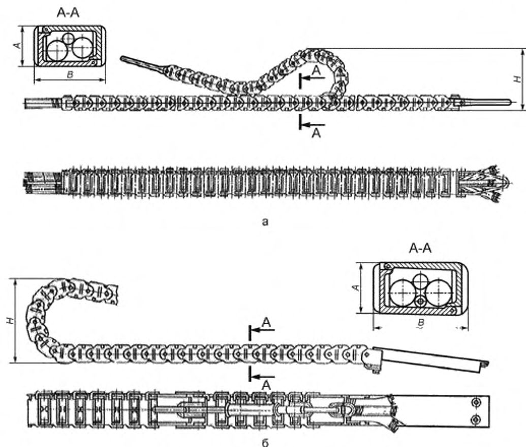
Рисунок 1 — Исполнение кабелеукладчика
