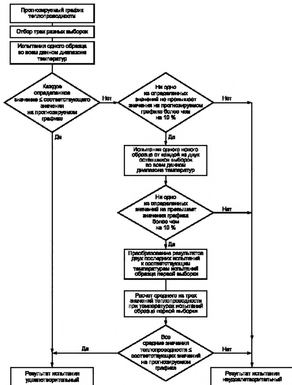
Рисунок 1 — Схема подтверждения теплопроводности
