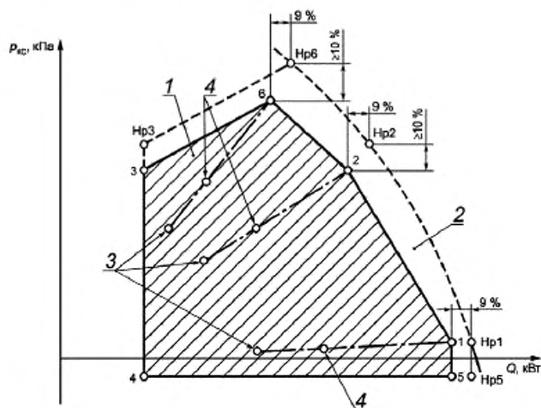
Рисунок 3 — Рабочая и испытательная диаграммы для одноступенчатой горелки (точки Нр3 и Нр5 не определены)
