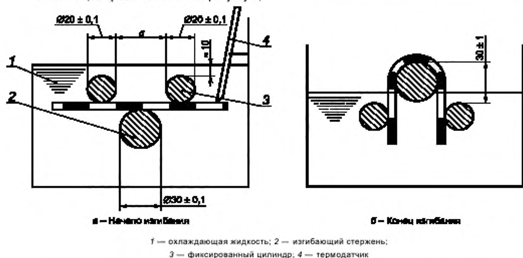
Рисунок 1 — Конструкция и принцип действия изгибающего приспособления
