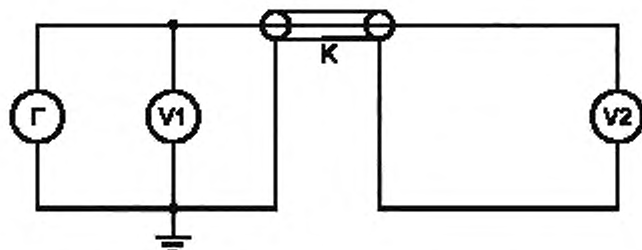
Г — генератор; V1, V2 — вольтметры; К — кабель
