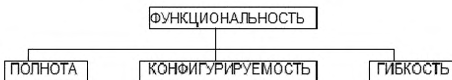
Рисунок 2 — Иерархия функциональности
