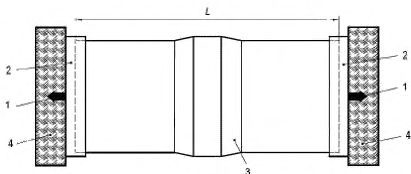
Рисунок 1 – Схема нагружения образцов при продольных нагрузках
