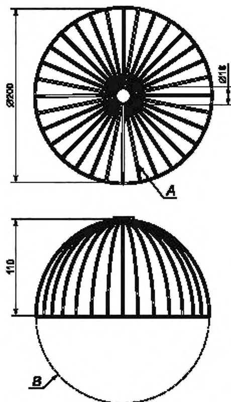
А — каркас из 32 равномерно расположенных проволок диаметром (1,5 \pm 0,5) мм; В — положение деревянной сферы
