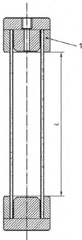
Рисунок 2 – Схема установки заглушек на образце, при испытании с осевой нагрузкой
