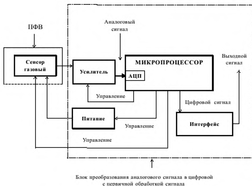
Рисунок 1 — Пример структурной схемы МЭГИ, включающего в себя блок ПФВ и блок преобразования аналогового сигнала в цифровой с первичной обработкой сигнала и введением корректировки в работу ПФВ по обратной
