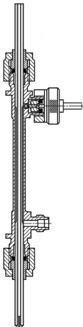
Рисунок А2.2 — Сборочный чертеж испытательной секции трубки нагревателя
