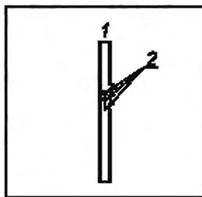
1 — испытываемая поверхность длиной 60 мм; 2 — примеры дефектов поверхности площадью 2,5 \text{ мм}^2 : квадрат, пятно, полоска шириной 0,8 мм
