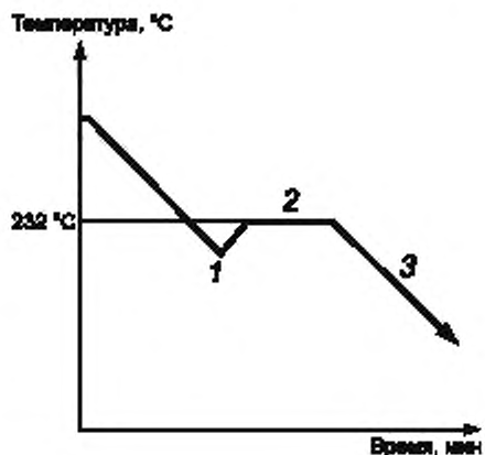
Рисунок А2.5 — Характеристика затвердевания олова
