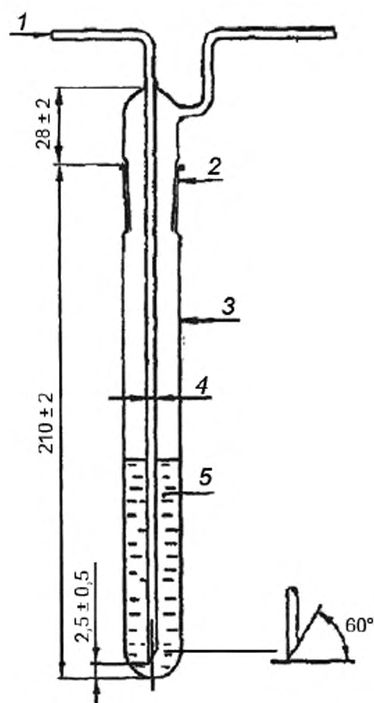
1 — подача воздуха или кислорода; 2 — конус В 24; 3 — наружный диаметр ( 28,0 \pm 0,5 ) мм, толщина стенки ( 1,4 \pm 0,2 ) мм, 4 — наружный диаметр ( 5,0 \pm 0,4 ) мм, толщина стенки ( 0,8 \pm 0,1 ) мм; 5 — изоляционная или абсорбирующая жидкость
