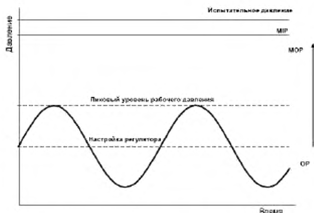
Рисунок 1 – Соотношение давлений
