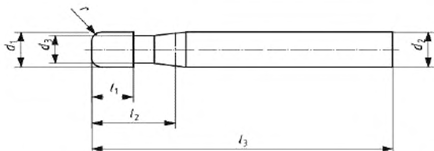
Рисунок 1 — Фрезы типов 1 и 2
