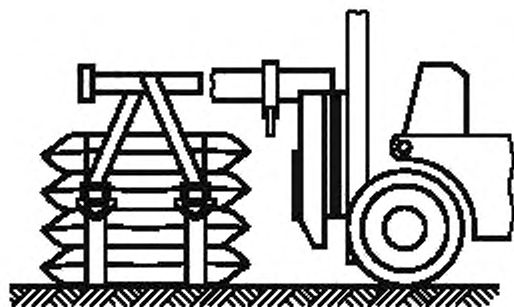
Рисунок 10 — Транспортировка груза погрузчиком со штыревым захватом
