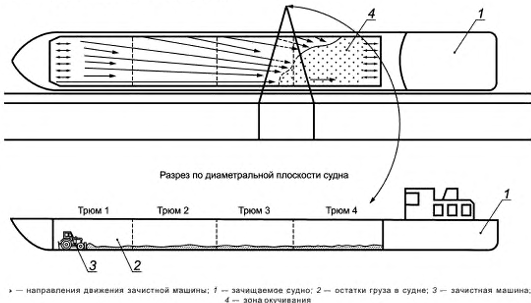
Рисунок 2 — Схема использования зачистной машины
