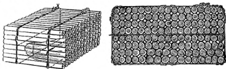
Рисунок 5 — Пакет круглого леса в полужестком строле
