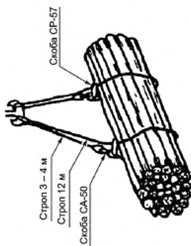
Перегрузка груза строповой подвешной
