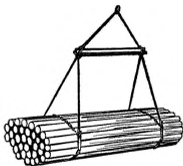
Рисунок 7 — Схема строповки длинномерного груза
