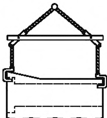
Рисунок 8 — Схема строповки железобетонной трубы
