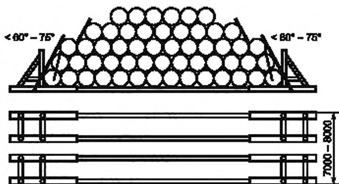
Рисунок 12 — Схема размещения груза на складе
