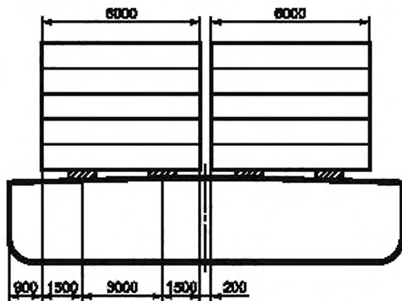
Рисунок 14 — Схема размещения груза в судне
