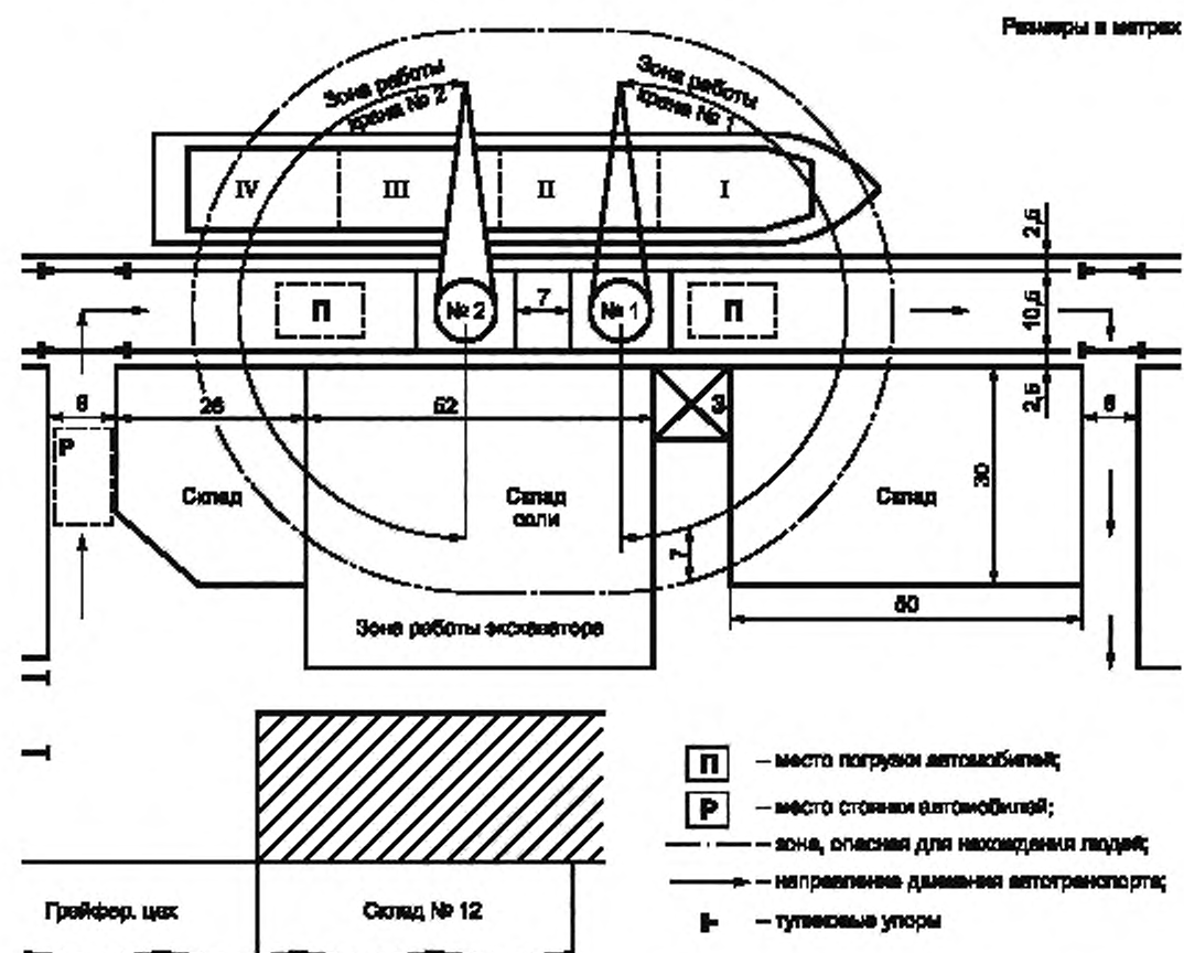
Рисунок 1 — Графическое изображение технологической схемы
