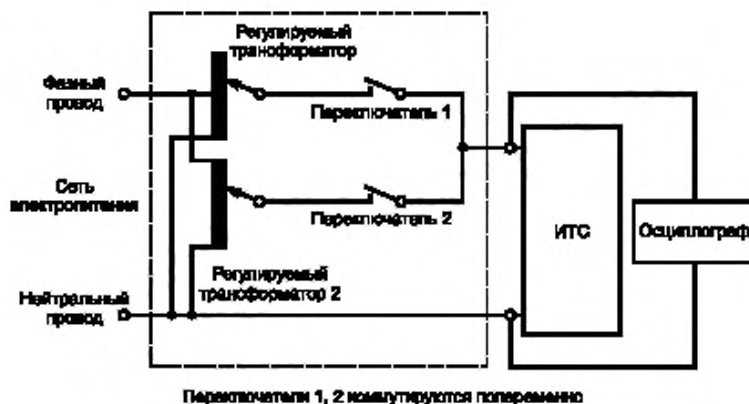
а) Схема испытаний с использованием регулировочных трансформаторов и переключателей
