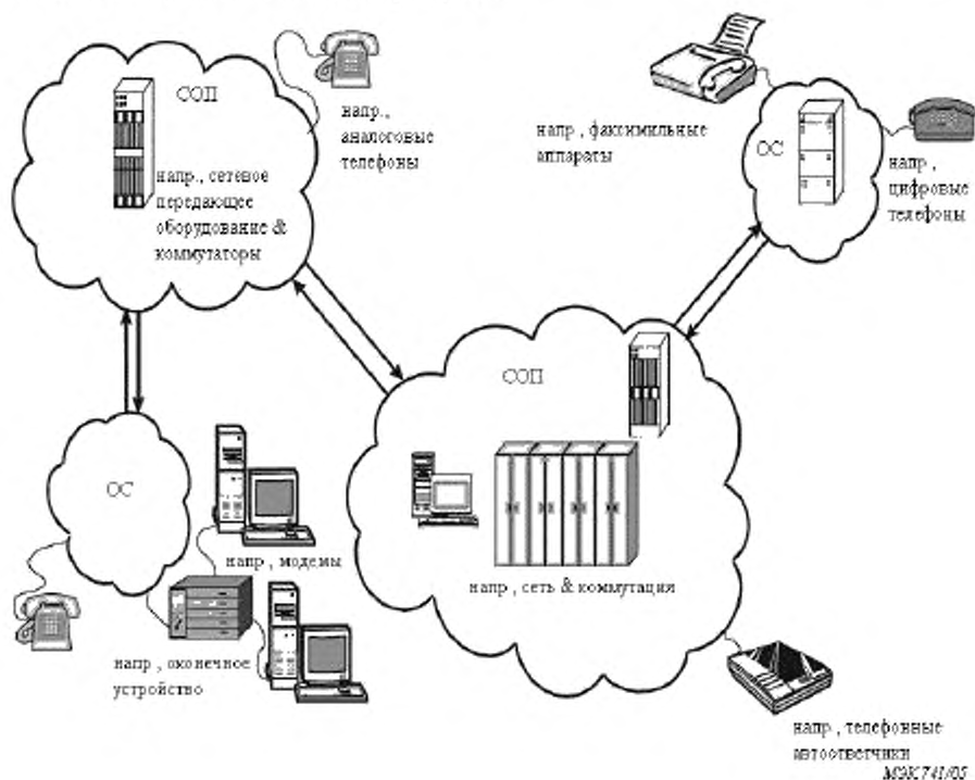
Рисунок 1 – Базовая конфигурация
