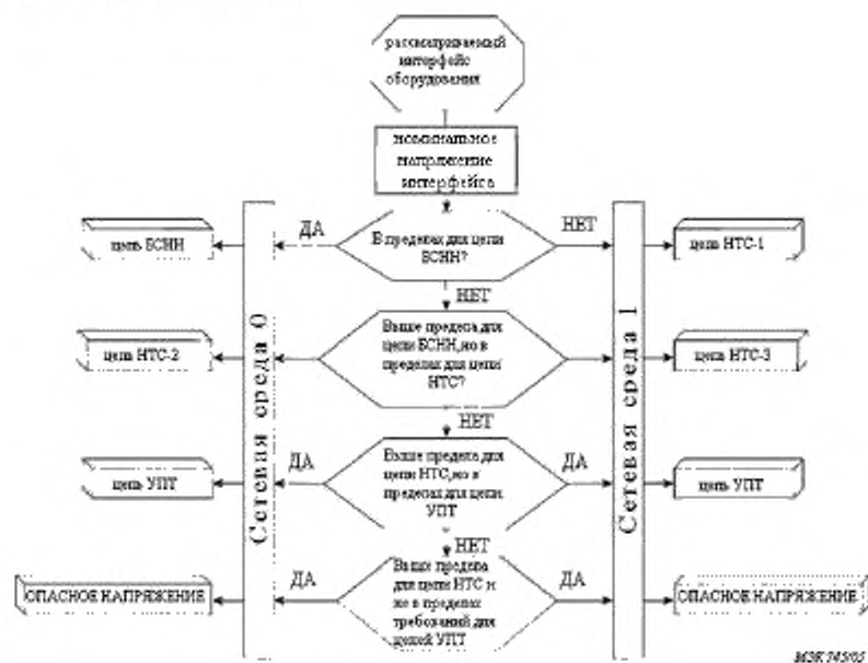
Рисунок 3 – Блок-схема для определения типа цепи
