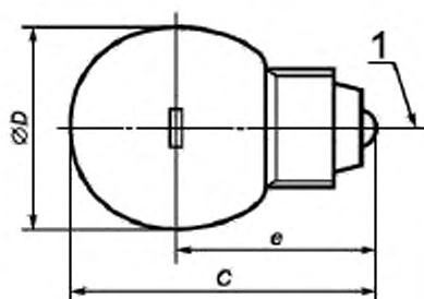
1 – базовая ось
