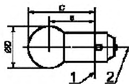
2 – базовая ось
