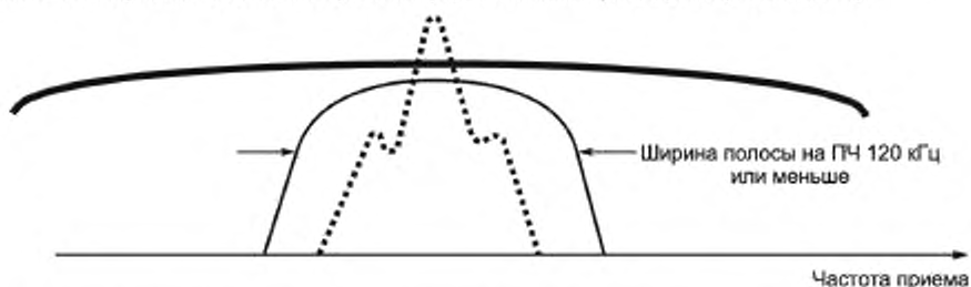
Рисунок A.9 — Амплитудно-модулированная ИРП от испытуемого ТС (пунктирная кривая)
