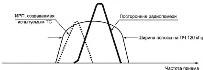
Рисунок А.3 — Немодулированная ИРП (пунктирная кривая)
