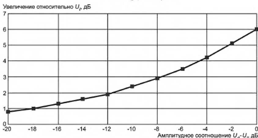
Рисунок А.10 — Увеличение пикового значения при суперпозиции двух немодулированных сигналов ( U_a — уровень посторонних радиопомех; U_i — уровень ИРП, создаваемых испытуемым ТС)
