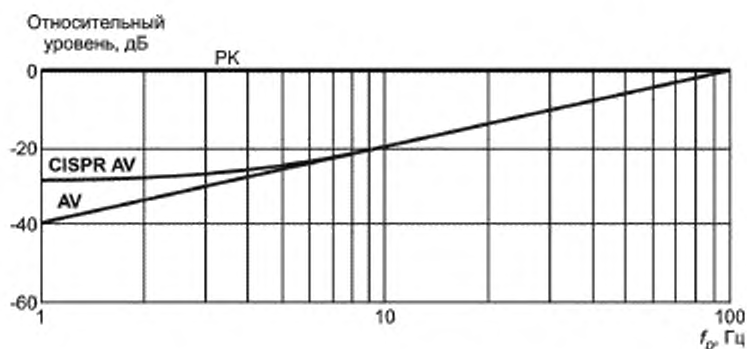
Рисунок D.2 — Весовая функция импульса 10 мс при детектировании пиковым детектором «ПК», детектором средних значений при учете пиковых значений «CISPR AV» и детектором средних значений без учета пиковых значений «AV» для постоянной времени прибора 100 мс
