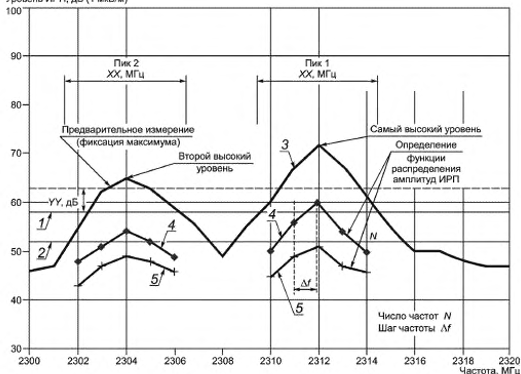
Рисунок Е.1 — Пример применения функции распределения амплитуд для флюктуирующих помех, метод 1
