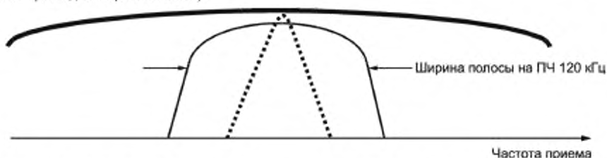
Рисунок A.8 — Немодулированная ИРП, создаваемая испытуемым ТС (пунктирная кривая)
