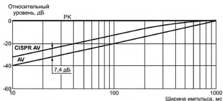
Рисунок D.3 — Пример весовых функций (импульс 1 Гц) при детектировании пиковым детектором «ПК» и детектором средних значений «AV» относительно ширины импульсов для постоянной времени прибора 160 мс
