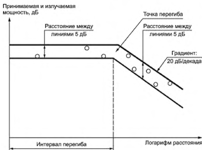
Рисунок 17 — Определение «интервала перегиба»
