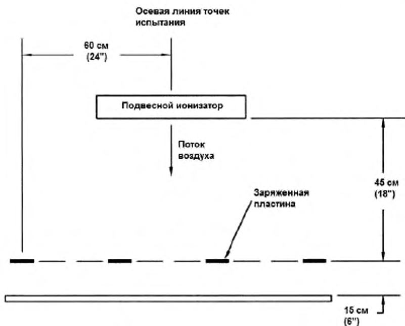
Рисунок 14. Области испытаний подвесного ионизатора (вид сбоку)
