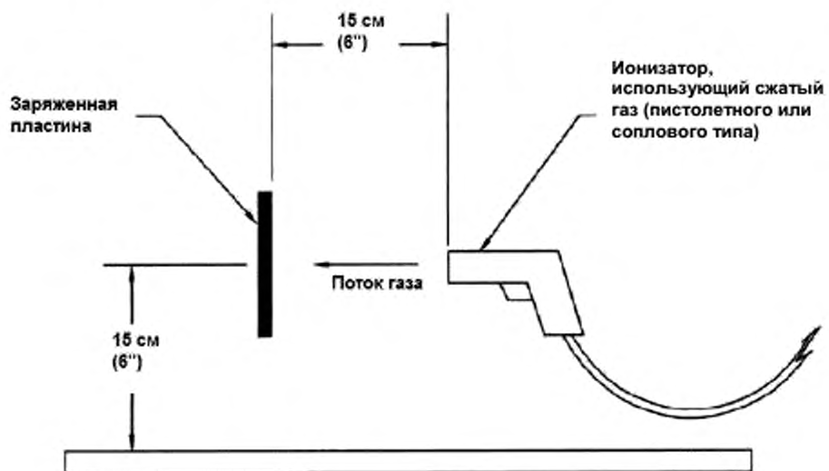
Рисунок 15. Области испытаний ионизатора, использующего сжатый газ (пистолетного или соплового типа) (вид сбоку)
