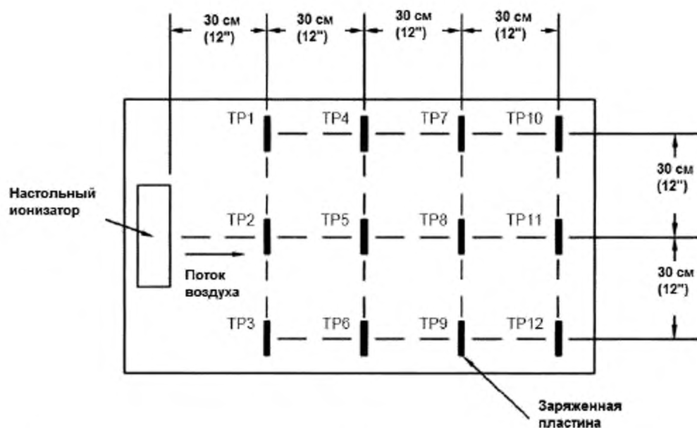
Рисунок 11. Области испытаний настольного ионизатора (вид сверху)
