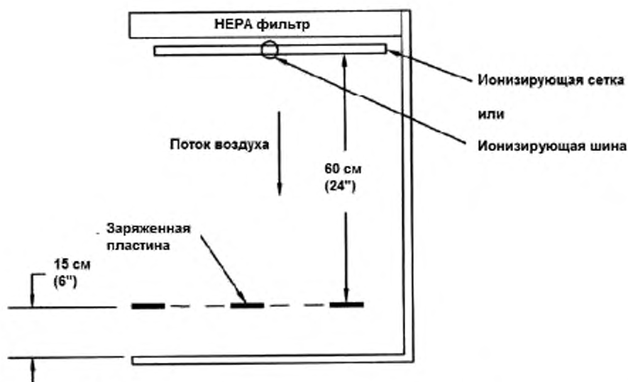
Рисунок 8. Области испытаний ионизации в направлении вертикального ламинарного потока воздуха (вид сбоку)
