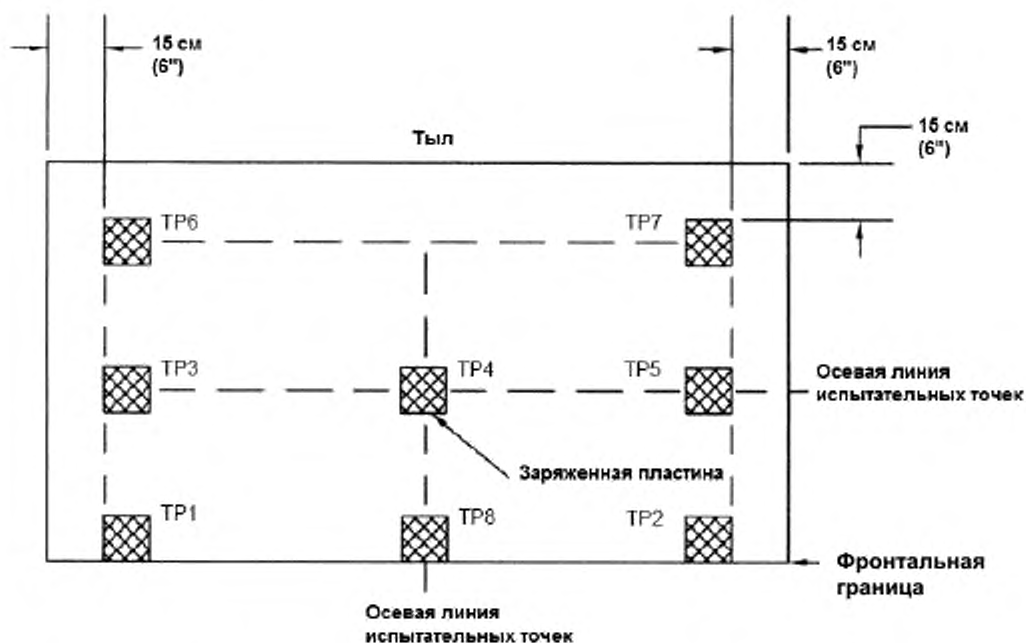
Рисунок 7. Области испытаний ионизации в направлении вертикального ламинарного потока воздуха (вид сверху)
