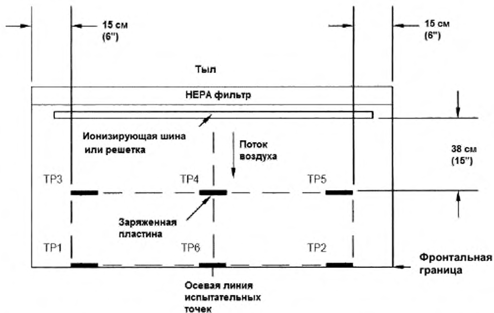
Рисунок 9. Области испытаний ионизации в направлении горизонтального ламинарного потока воздуха (вид сверху)
