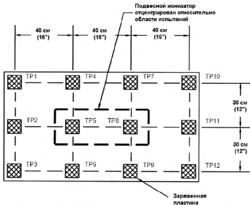
Рисунок 13. Области испытаний подвесного ионизатора (вид сверху)
