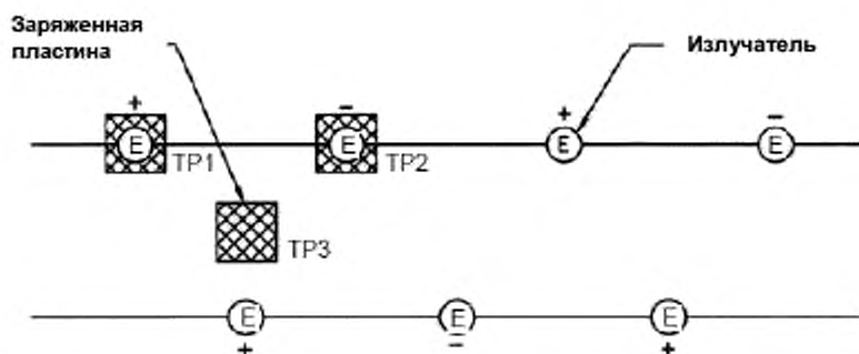
Рисунок 5. Области испытаний ионизации всего помещения. Системы двойных линий постоянного тока
