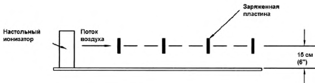
Рисунок 12. Области испытаний настольного ионизатора (вид сбоку)
