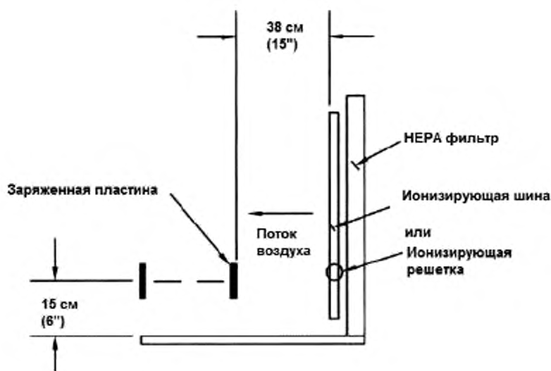
Рисунок 10. Области испытаний ионизации в направлении горизонтального ламинарного потока воздуха (вид сбоку)
