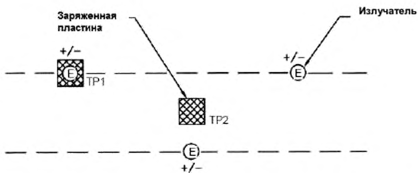
Рисунок 6. Области испытаний ионизации всего помещения. Системы излучателей постоянного тока переменной полярности
