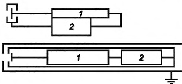
1 — электростатический вольтметр; 2 — обратная связь
