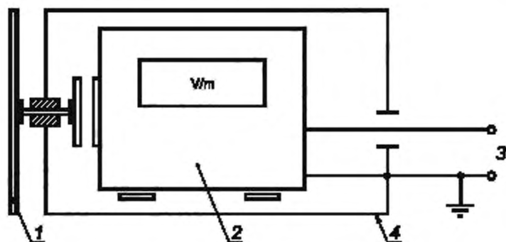
1 — изолированный электрод; 2 — измеритель поля; 3 — внешний выход; 4 — экран
