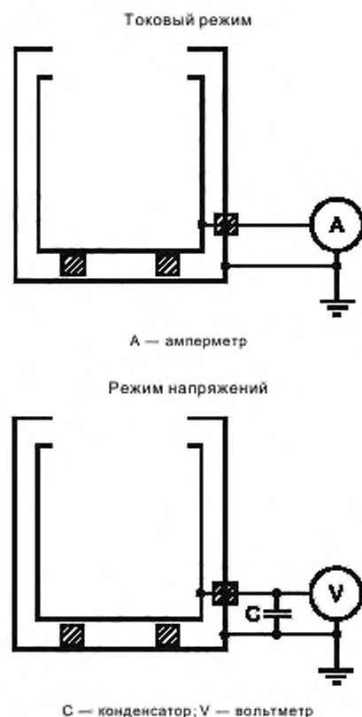
Рисунок 2 — Схемы измерений заряда
