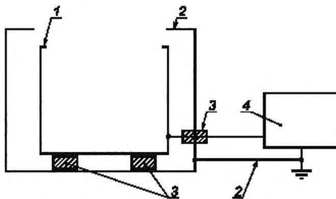
1 — внутренний контейнер; 2 — экран; 3 — изолятор; 4 — детектор
