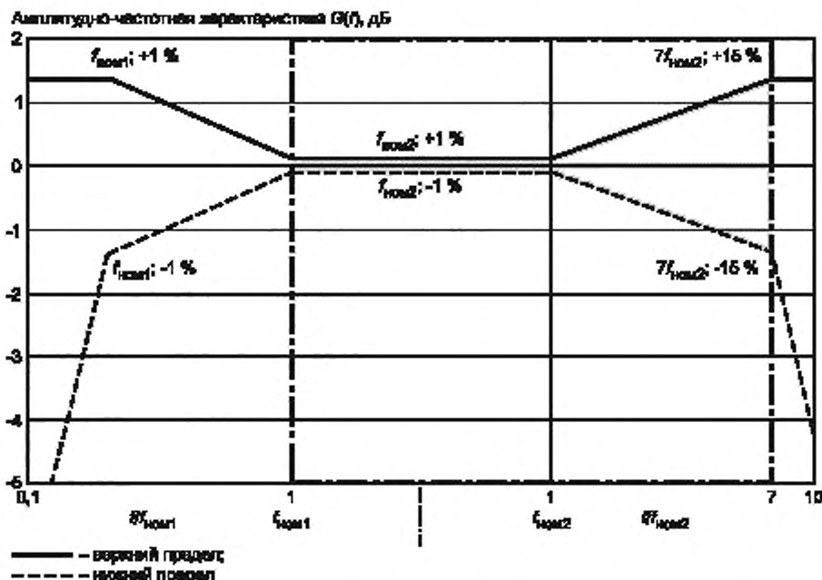
Рисунок 7 — Приемлемая нормализованная амплитудно-частотная характеристика измерительной системы (затемненная область), предназначенная для диапазона основных частот от f_{ном1} до f_{ном2} (испытанная в диапазоне f_{ном1}—7f_{ном2} )
