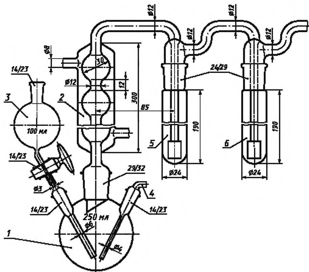
1 — дистилляционная колба; 2 — обратный холодильник; 3 — каплевая воронка; 4 — подводящая трубка; 5 и 6 — газопоглощающие устройства
